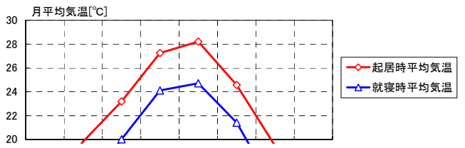
図3 平均気温
