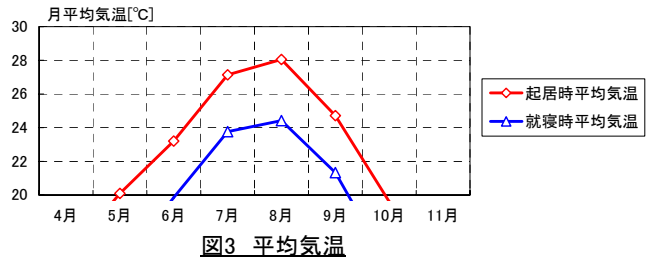
図3 平均気温
