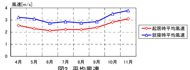
図2 平均風速
