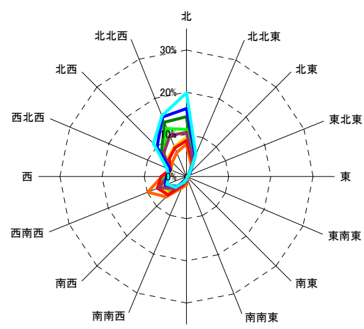
図4b 月別風配図(就寝時)
